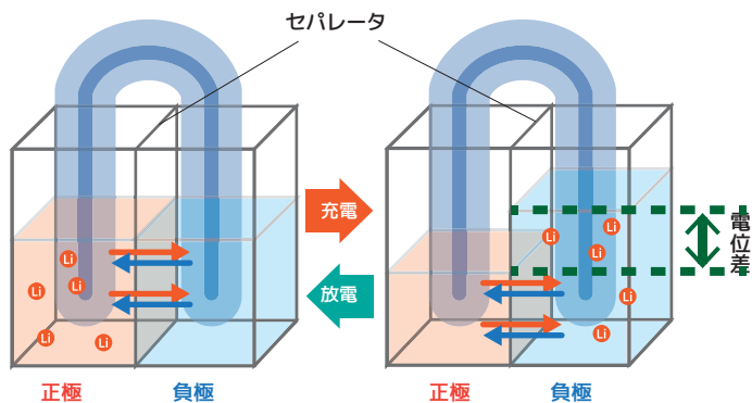
【電池原理】
